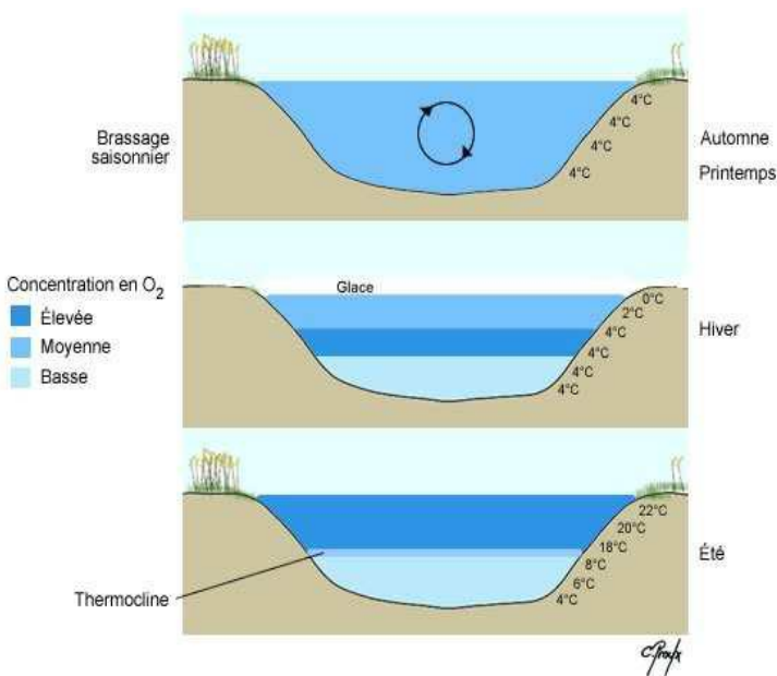
Figure 1 : Stratification thermique d'un lac dimictique † Source : Proulx, 2009
