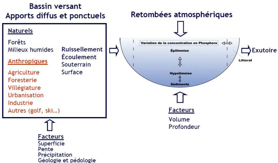
Figure 1 : Schéma illustrant le concept général de l'eutrophisation d'un plan d'eau et les apports du phosphore du bassin versant jusqu'au lac, qu'ils soient d'origine anthropique ou naturelle. Figure tirée de Roy, 2010.
